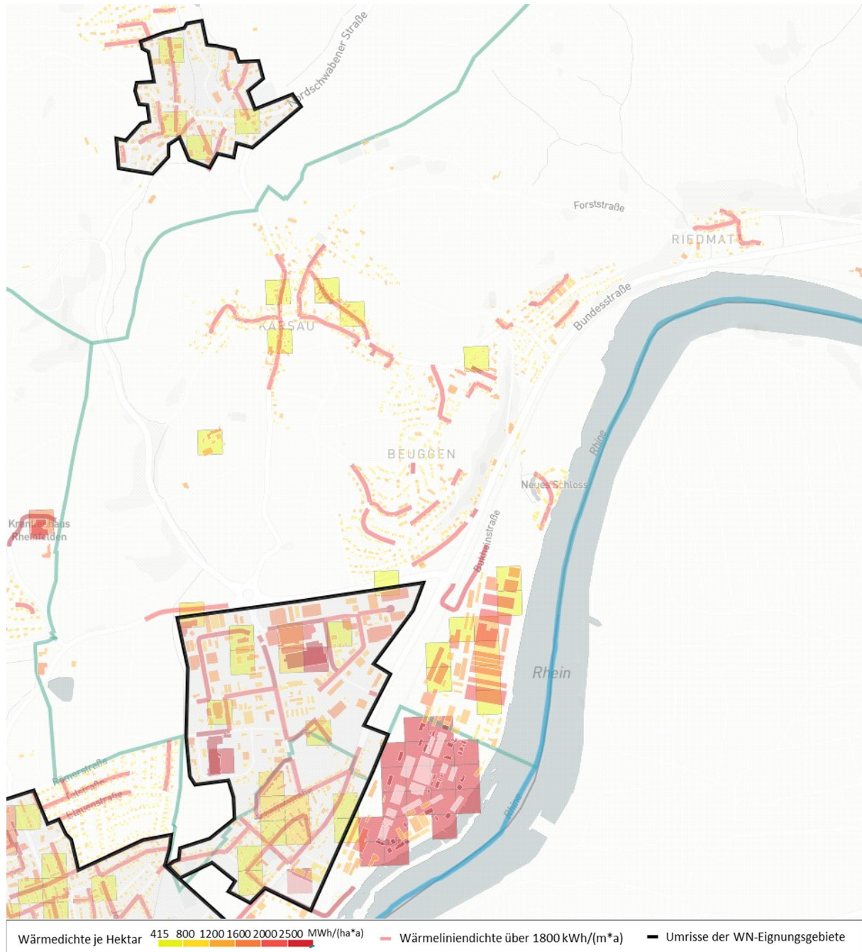
Abbildung 3: Gebiete mit hoher Wärmedichte (ab 415 MWh/ha) und Wärmenetz-Eignungsgebiete. Die hier dargestellte Wärmedichte stellt die Summe des gesamten Wärmeverbrauchs aller in einem Hektar (100 x 100 m) liegenden Gebäude dar. Je höher dieser Wärmeverbrauch ist, umso mehr verändert sich die Farbe von gelb nach Rot.
