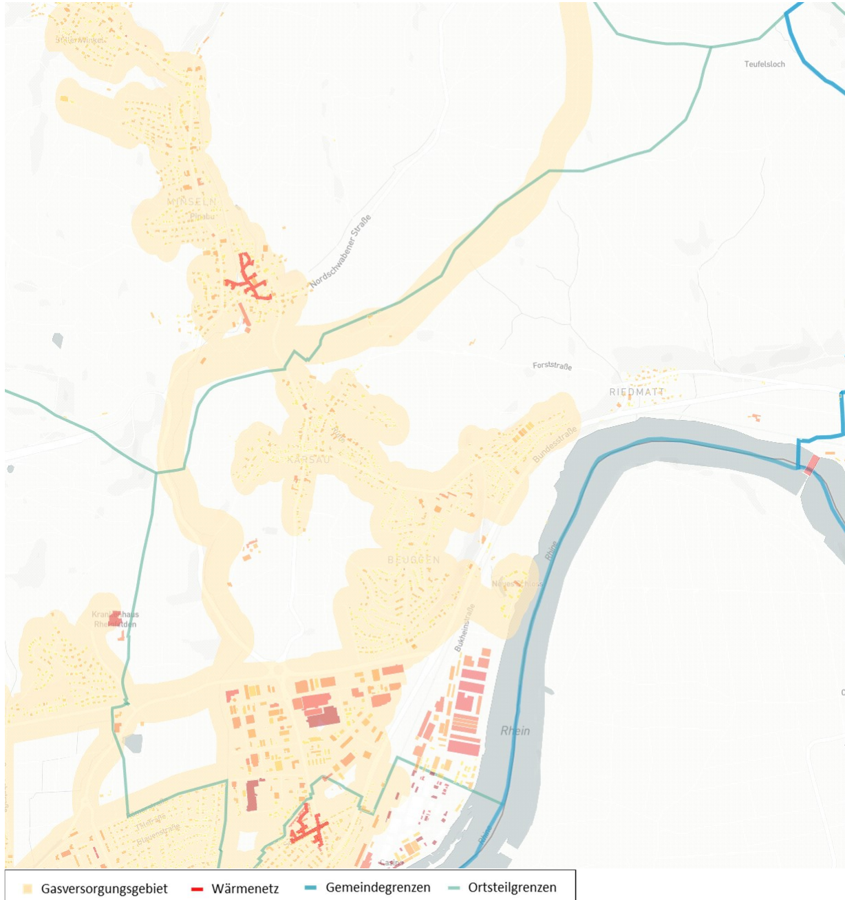
Abbildung 2: Vorhandene Wärme-Infrastruktur. Die Gebäude sind gemäß ihrem Wärmeverbrauch eingefärbt: Je höher dieser ist, umso mehr verändert sich die Farbe von gelb nach rot.
