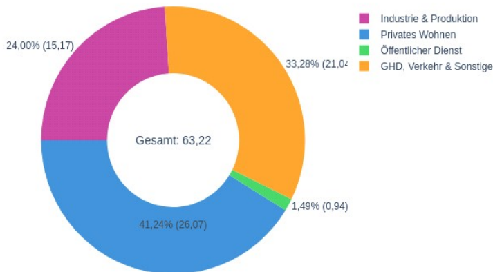
Wärmebedarf (in GWh/a) nach ökonomischen Sektoren
