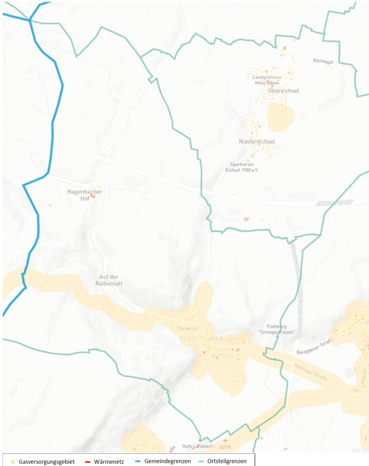
Abbildung 2: Vorhandene Wärme-Infrastruktur. Die Gebäude sind gemäß ihrem Wärmeverbrauch eingefärbt: Je höher dieser ist, umso mehr verändert sich die Farbe von gelb nach rot.
